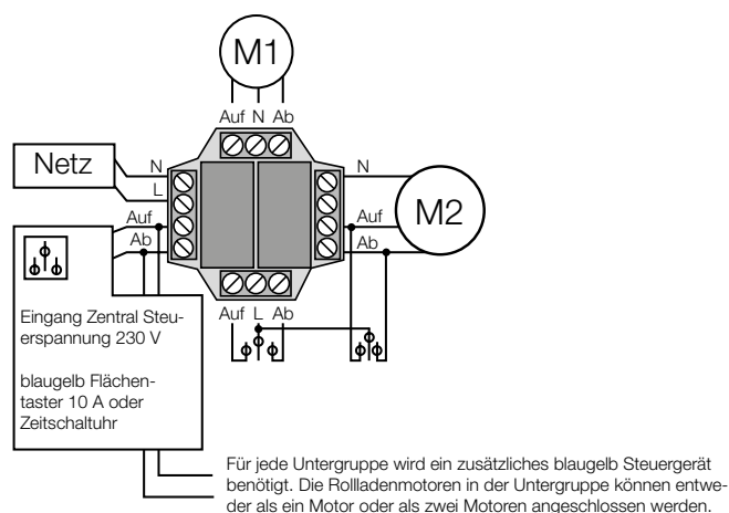
Anschlussplan für zwei Rollladenmotoren
