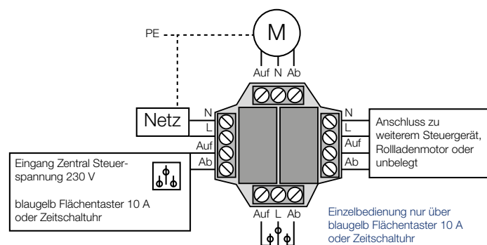
Anschlussplan für einen Rollladenmotor
